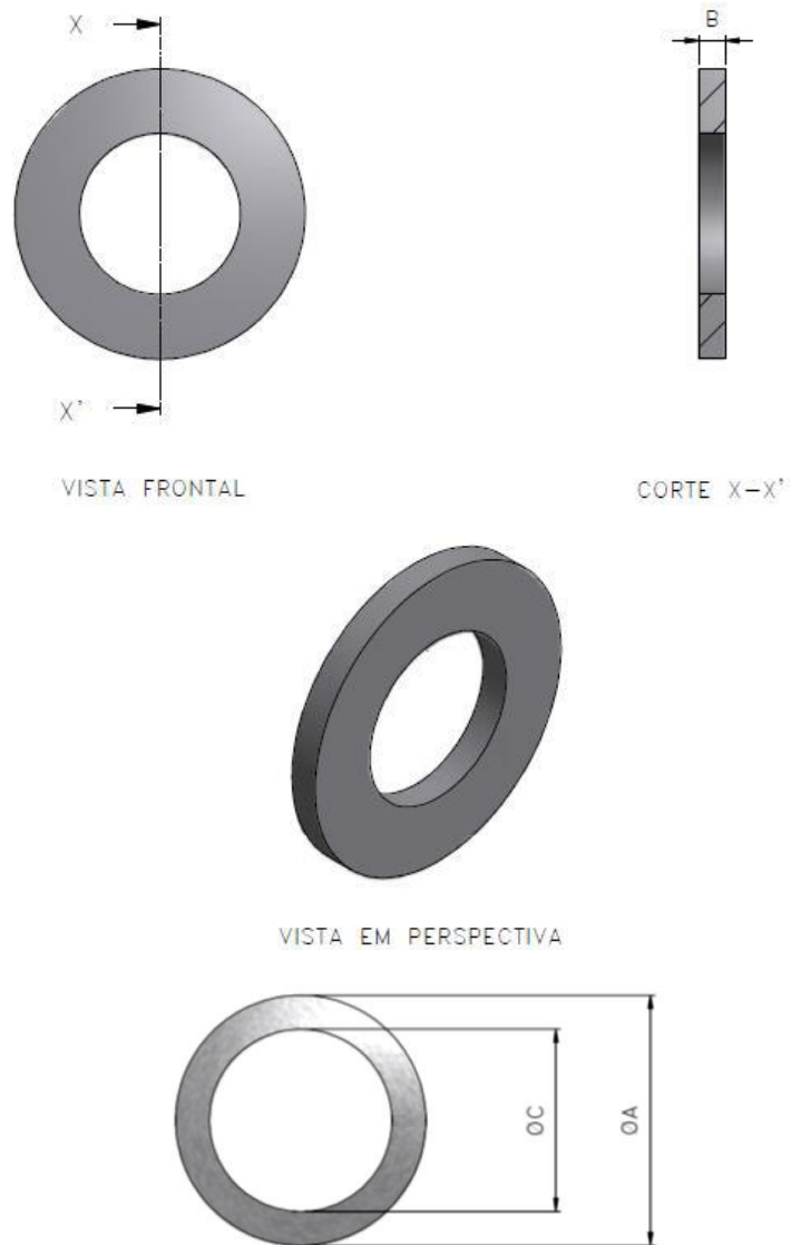
Figura 1 - Arruela Redonda - Liga de Alumínio
